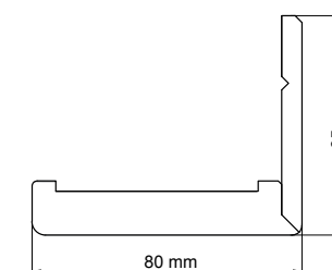
Kątownik poszerzający do ościeżnicy regulowanej - szerokość 80 mm
