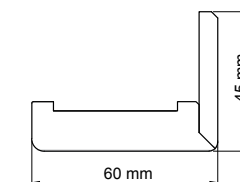
Kątownik do ościeżnicy regulowanej - szerokość 60 mm
